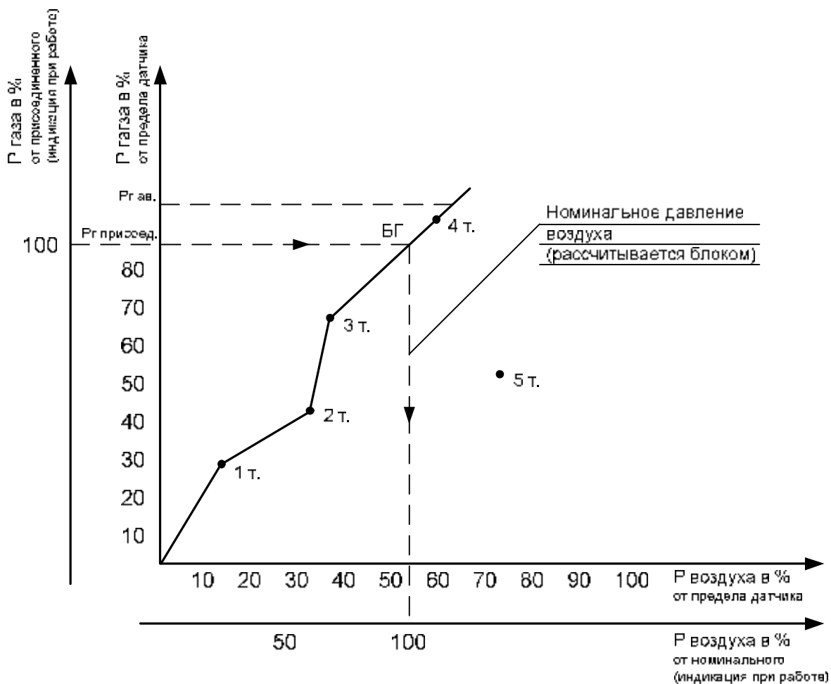
Рисунок 4. График соотношения топливо-воздух.
