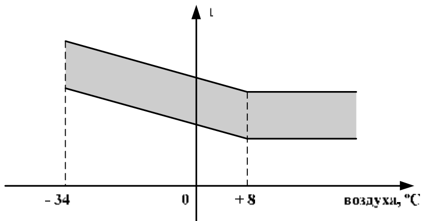
Рисунок 3. График зависимости температуры воды на выходе из котла от температуры наружного воздуха.
