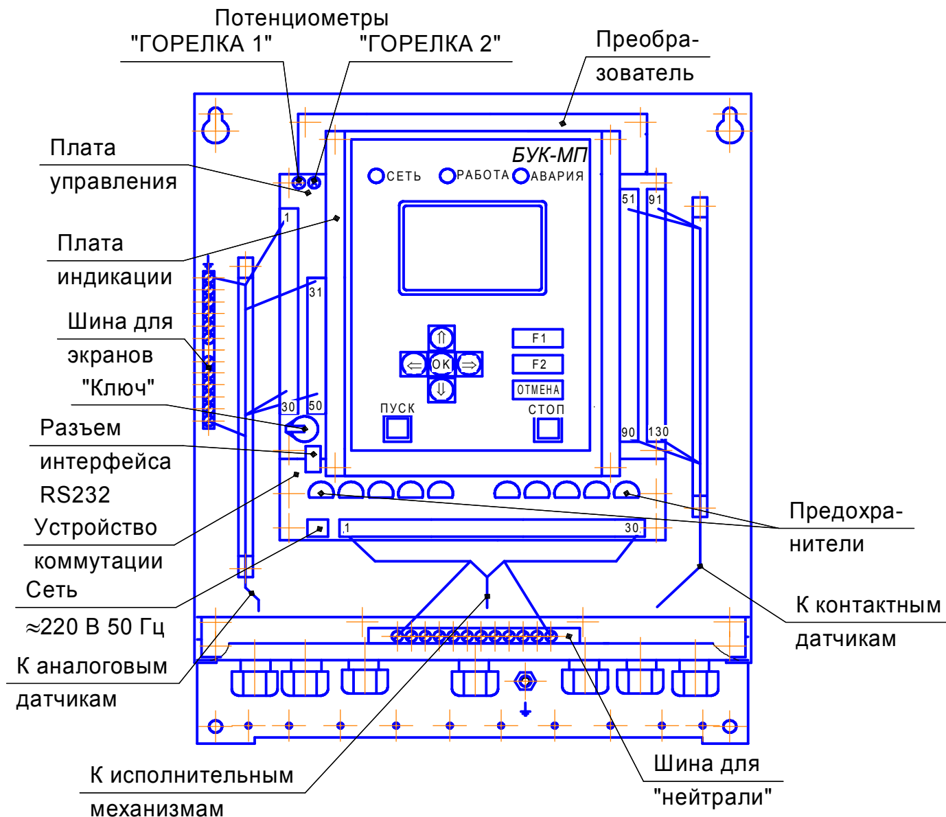
Рис. 2. Расположение разъемов на платах.
