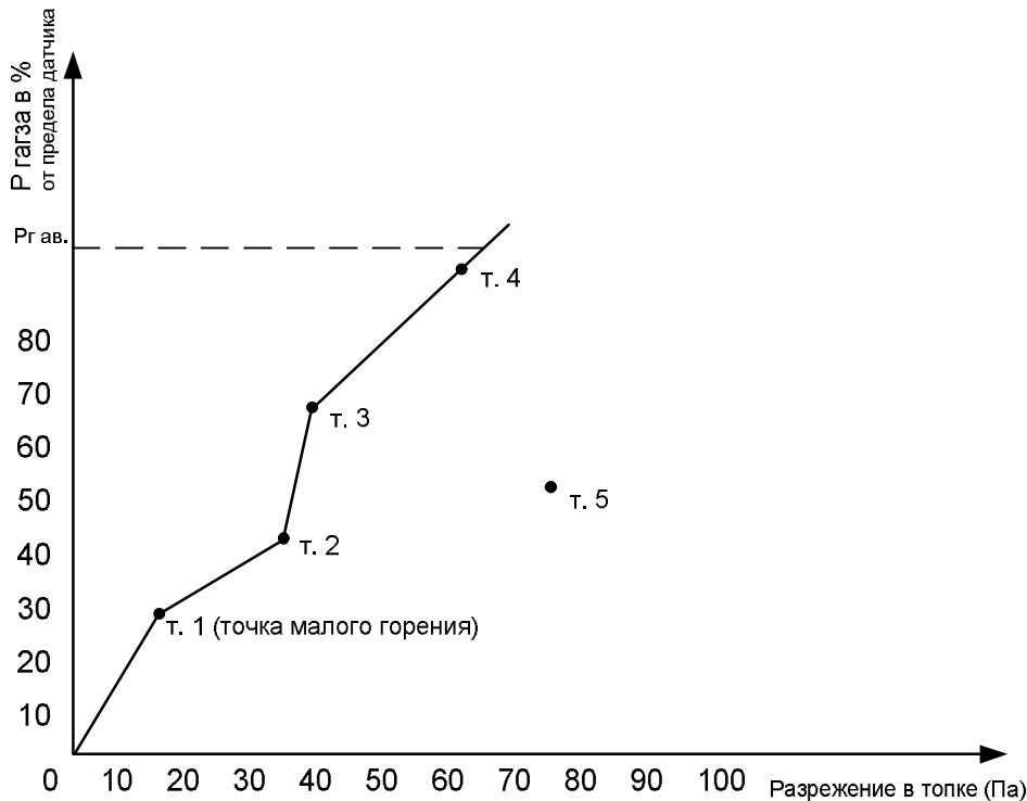
Рис. 3. График соотношения топливо-разрежение.
