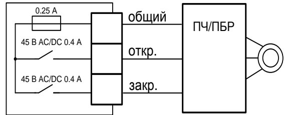
Управление 3-х фазным МЭО или частотным преобразователем
